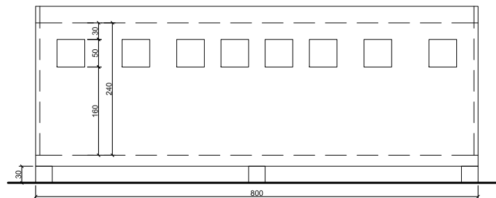
PROSPETTO RETRO MODULE 02, 1:50
