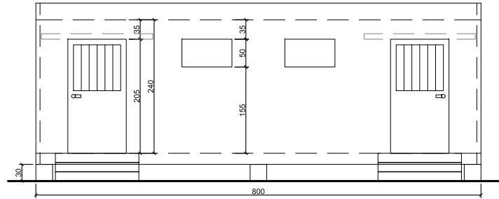
PROSPETTO PRINCIPALE MODULO 02, 1:50
