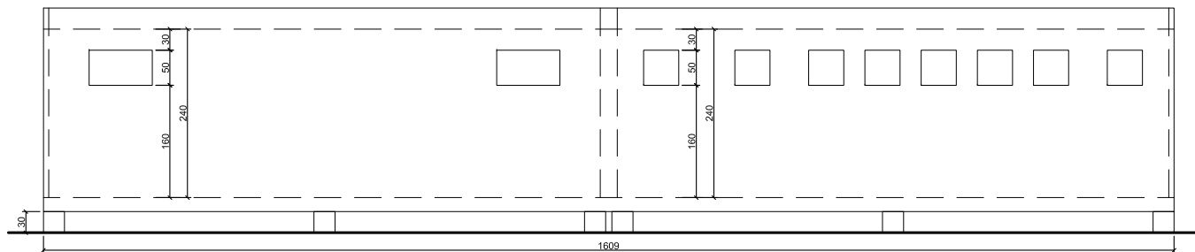
PROSPETTO RETRO MODULO 01, 1:50
