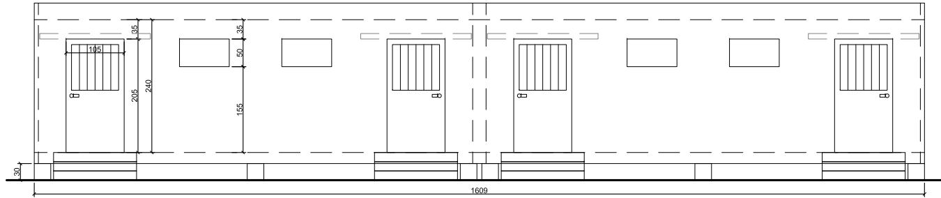
PROSPETTO PRINCIPALE MODULO 01, 1:50
